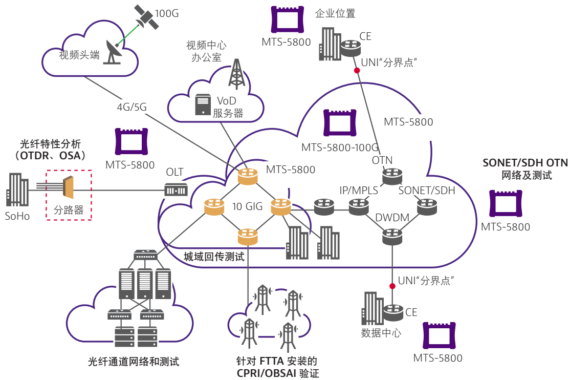
图 1. 运营商以太网中的 MTS-5800
